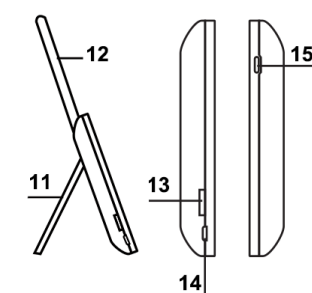
11. Standard (faltbar) 12. Antenne (faltbar) 13. Micro-SD-Karte 14. Micro-USB-Anschluss für Ladegerät 15. Ein-/Aus-Taste - kurz: Standby, lang (10 Sek.): alles aus 16. Mikrofon 17. Regenhaube und Türklingelhalter 18. Kamera 19. PIR-Bewegungssensor 20. Klingeltaster mit LED-Ring 21. Pairing-Taste 22. Stromanschluss 8-36V DC & 8-24V AC 23. Schraubenlöcher für die Wandmontage 24. Herausnehmbare und wiederaufladbare Akku 3,7V 5000 mAh 25. Lautsprecher 26. USB-C -Anschluss für Ladegerät
