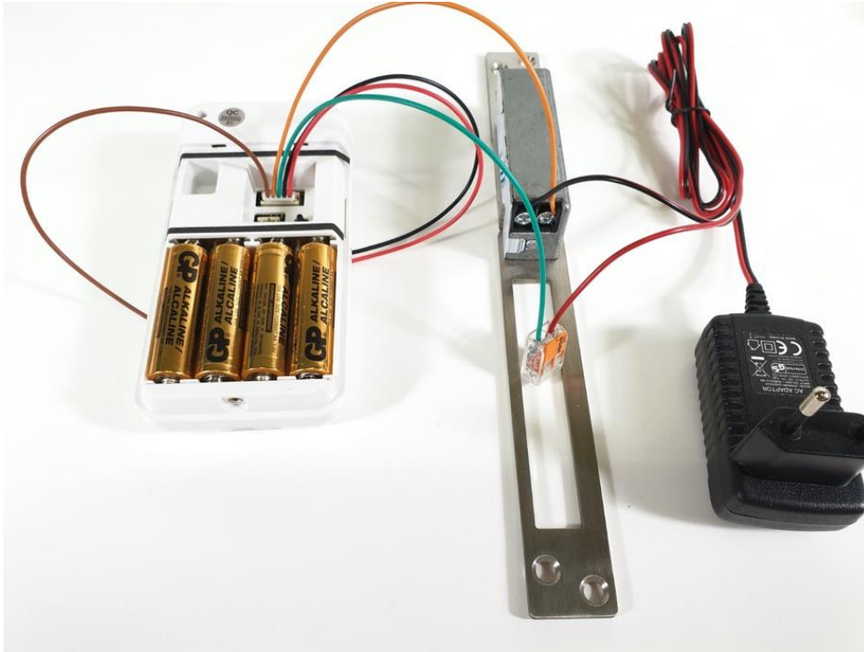
N.C. - Betriebsstrom
